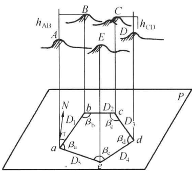
图 1-5 确定地面点位
