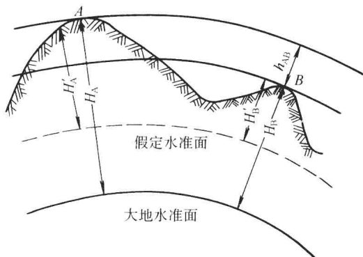
图 1-3 大地水准面
