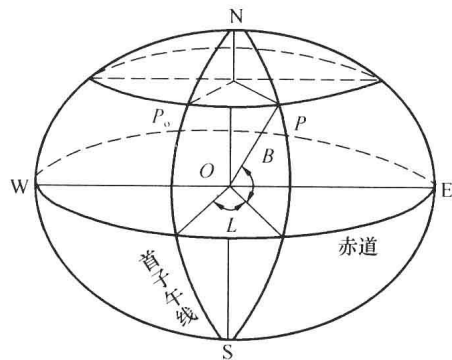
图 1-2 大地坐标
