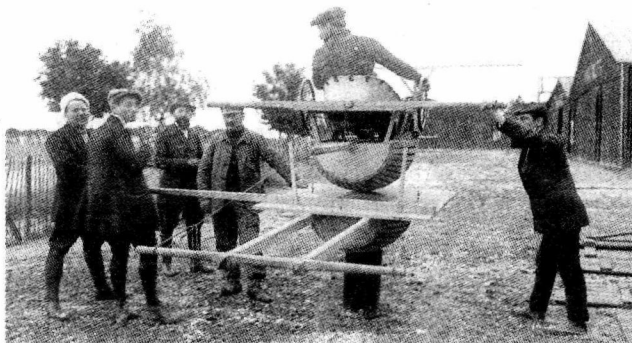
图 1-1 使用木桶、铁环与木头支架做成的飞行模拟器
