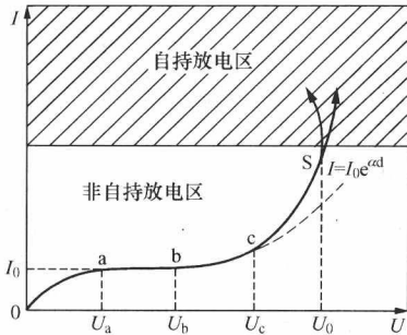
图 1-3 气体放电的伏安特性曲线
