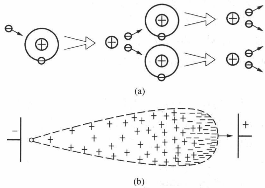
图 1-4 电子崩示意图
