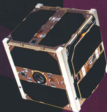
瑞士立方体卫星
