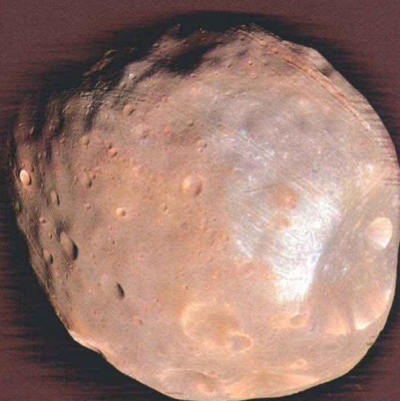
火卫一
