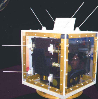
希望号卫星
