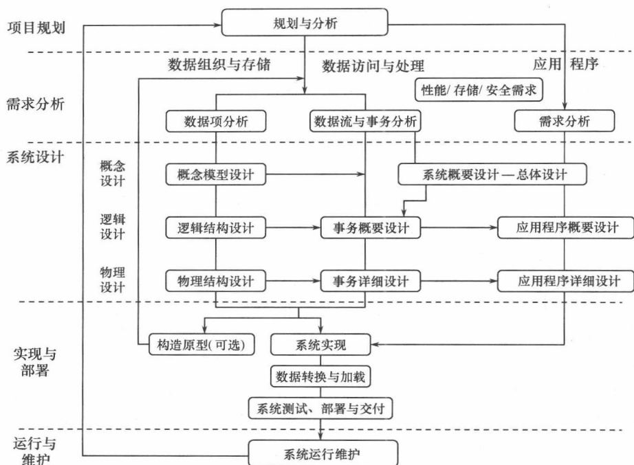
图 1.1 数据库应用系统生命周期模型
