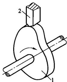
图 1-5 高副 1,2—构件
