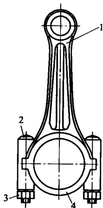
图 1-1 连杆
