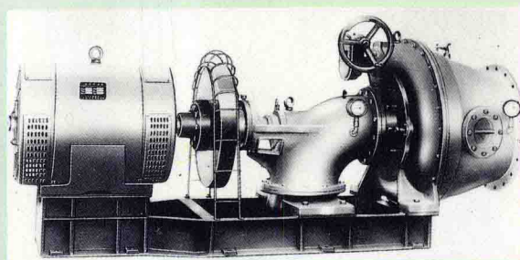
县水电设备厂参加西德汉诺威国际博览会的HL310系列混流式水轮发电机组
