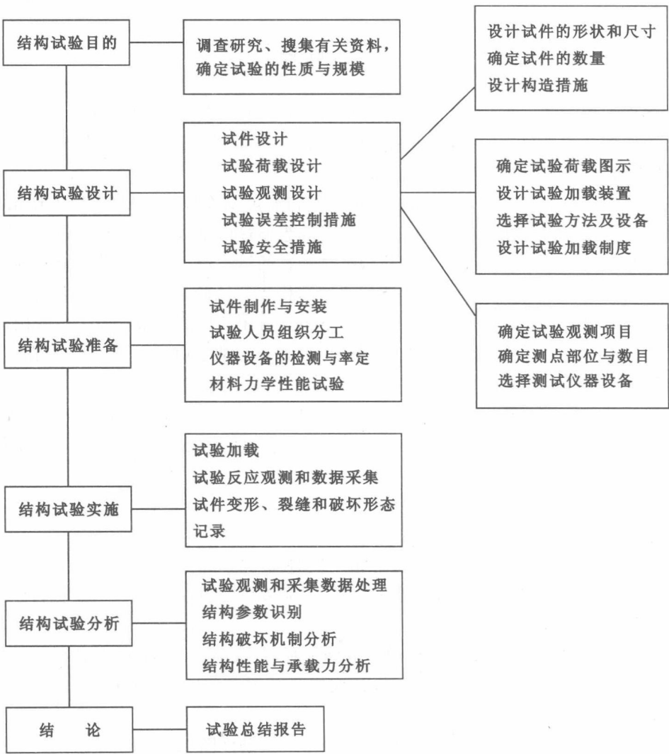
图 1.1 结构试验总框图
