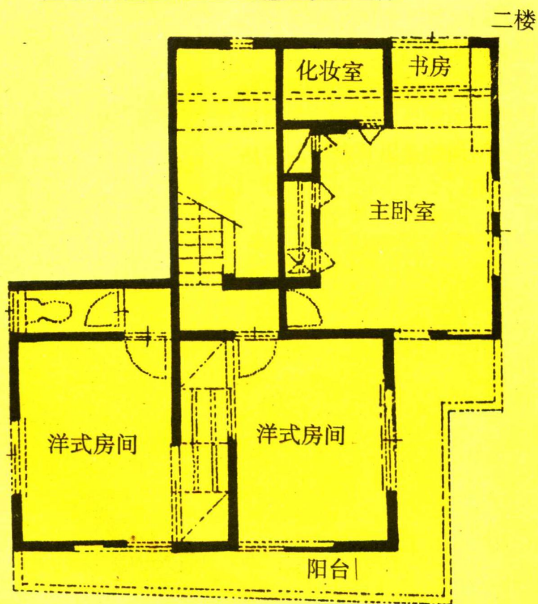
建筑平面图
