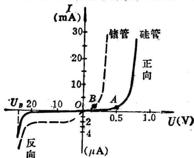
图 9-8 二极管的伏安特性曲线
