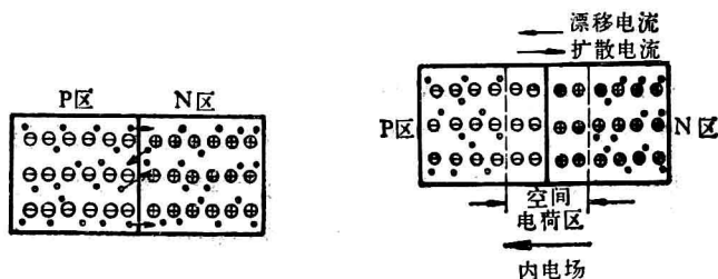
图9-4 PN结中载流子的扩散运动
