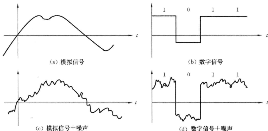
图 1-8 模拟信号与数字信号分别加入噪声的前后对比
