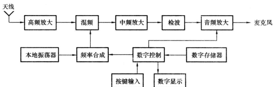
图 1-2 普通调幅收音机方框图
