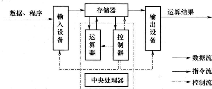
图 1-4 计算机硬件系统结构图
