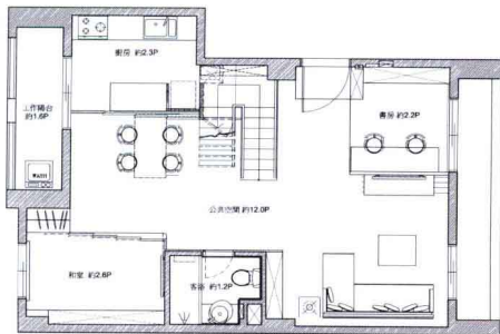
1F平面配置图
