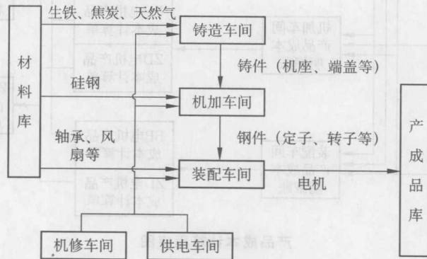
生产工艺流程图
