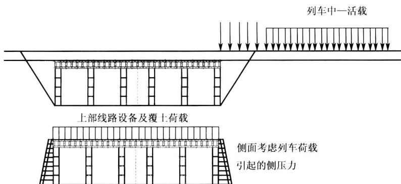
图2—7 工况1 荷载布置图
