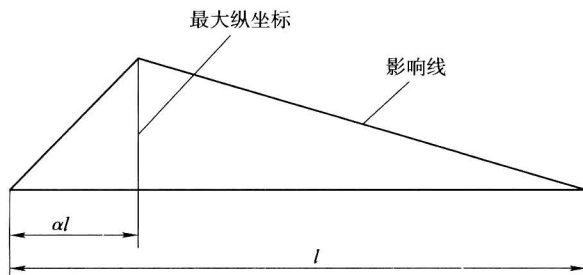
图 2—5 影响线
