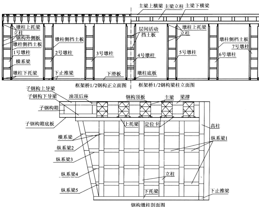
图2—1 主盾构体
