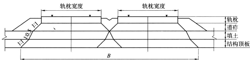
图 2—4 双线或多线顶桥活载分布
