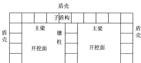
图 1—1 框架桥盾构横断面图
