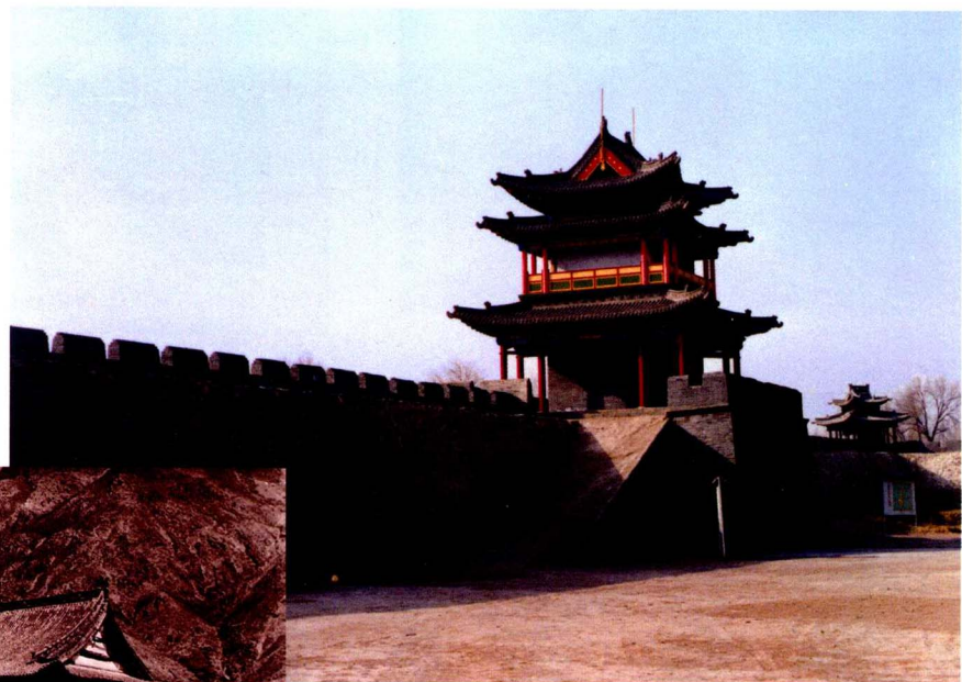
5—7 美岱召城楼及马道
