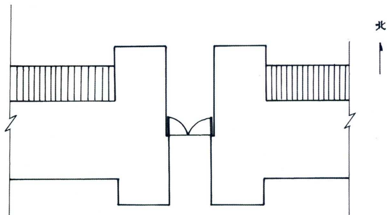
5—5 美岱召城门洞平面图
