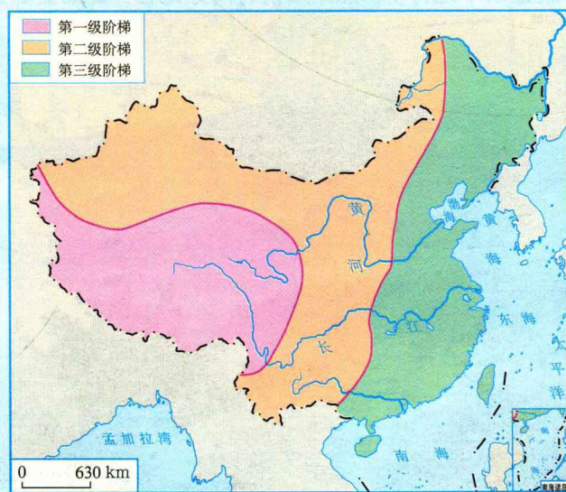
图 7.6 中国地势三级阶梯示意图
