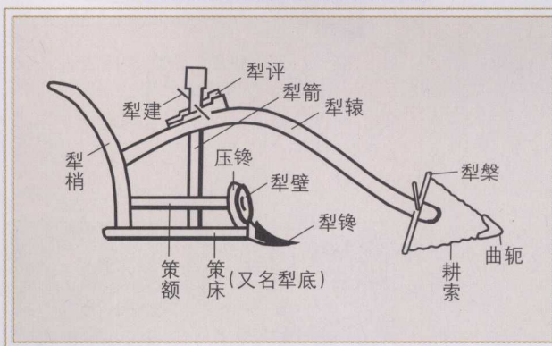
曲辕犁构造示意图
