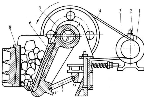
图 0.2 颚式破碎机
