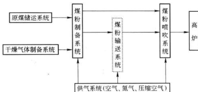
图 1-1 高炉喷煤系统的工艺流程
