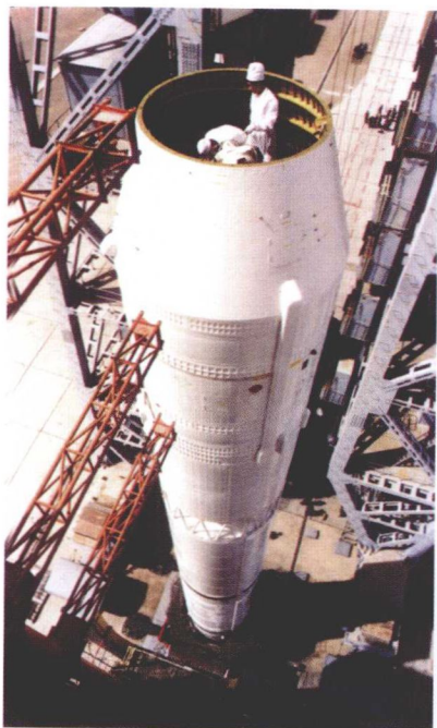
发射中队操作人员在长征二号运载火箭的仪器舱内安装陀螺平台。
