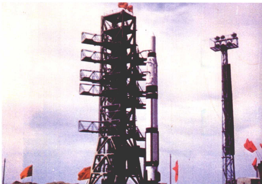
整装待发的东方红一号卫星和长征一号运载火箭。
