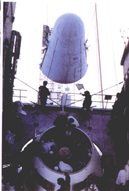
发射中队操作人员在长征二号运载火箭的仪器舱内安装陀螺平台。
