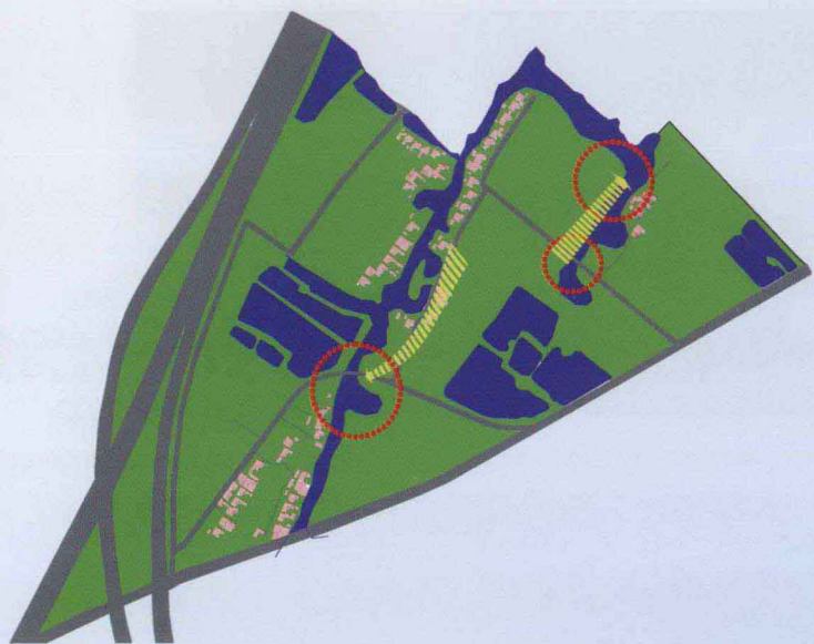
图16 董浜镇水稻区景观总体布置图
