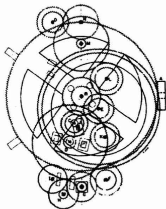
安蒂基西拉机器内部结构复原图
