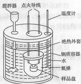
图 1-1 弹式量热计
