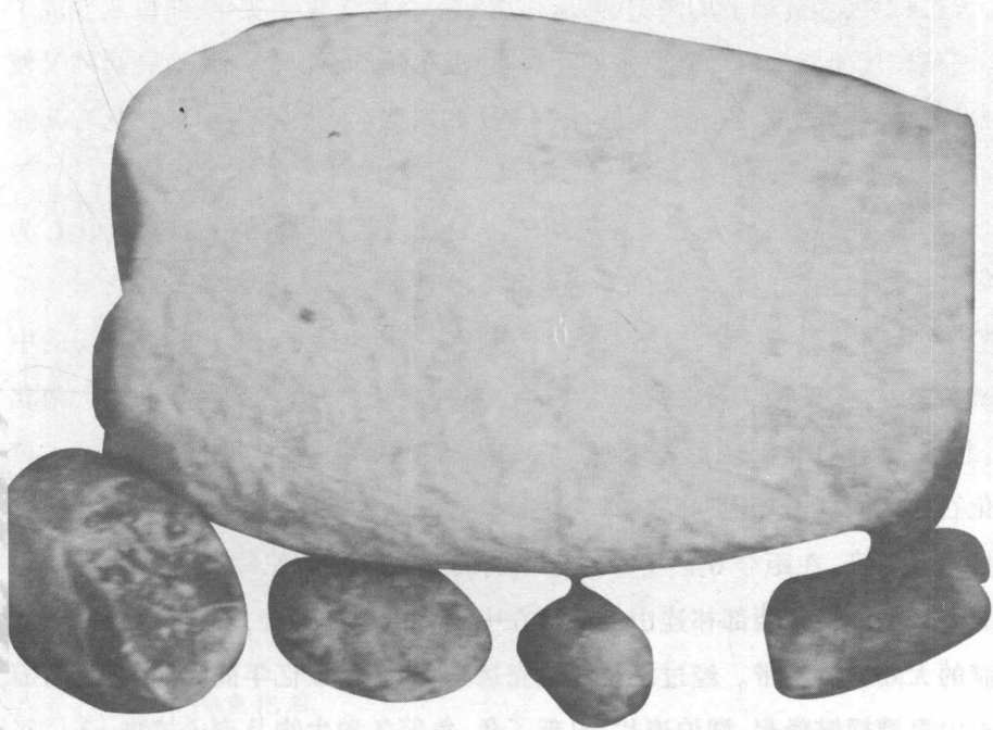
平塘湖植物果实化石
