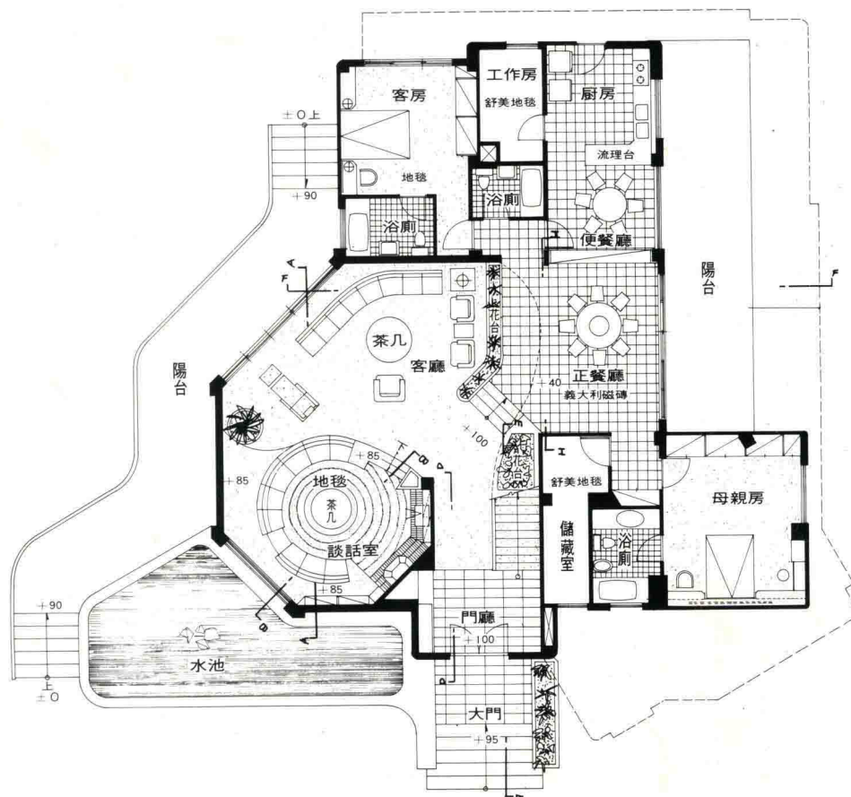
一樓平面圖
