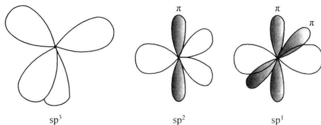
图 1.1 碳的成键类型 [6]
