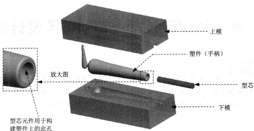
图 1.1.2 塑件成型元件 (带型芯)
