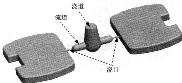
图 1.1.4 浇注系统
