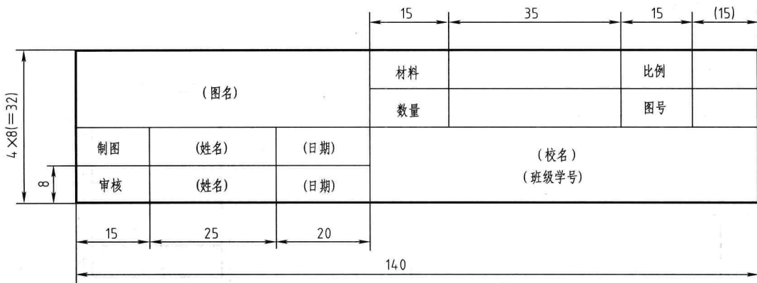
图 1-4 制图作业中推荐的标题栏格式
