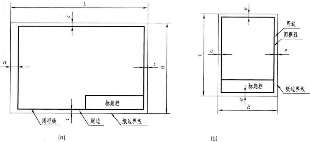
图 1-2 图框格式
