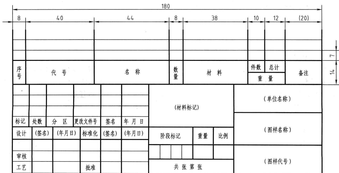
图 1-5 明细栏的格式(参考)
