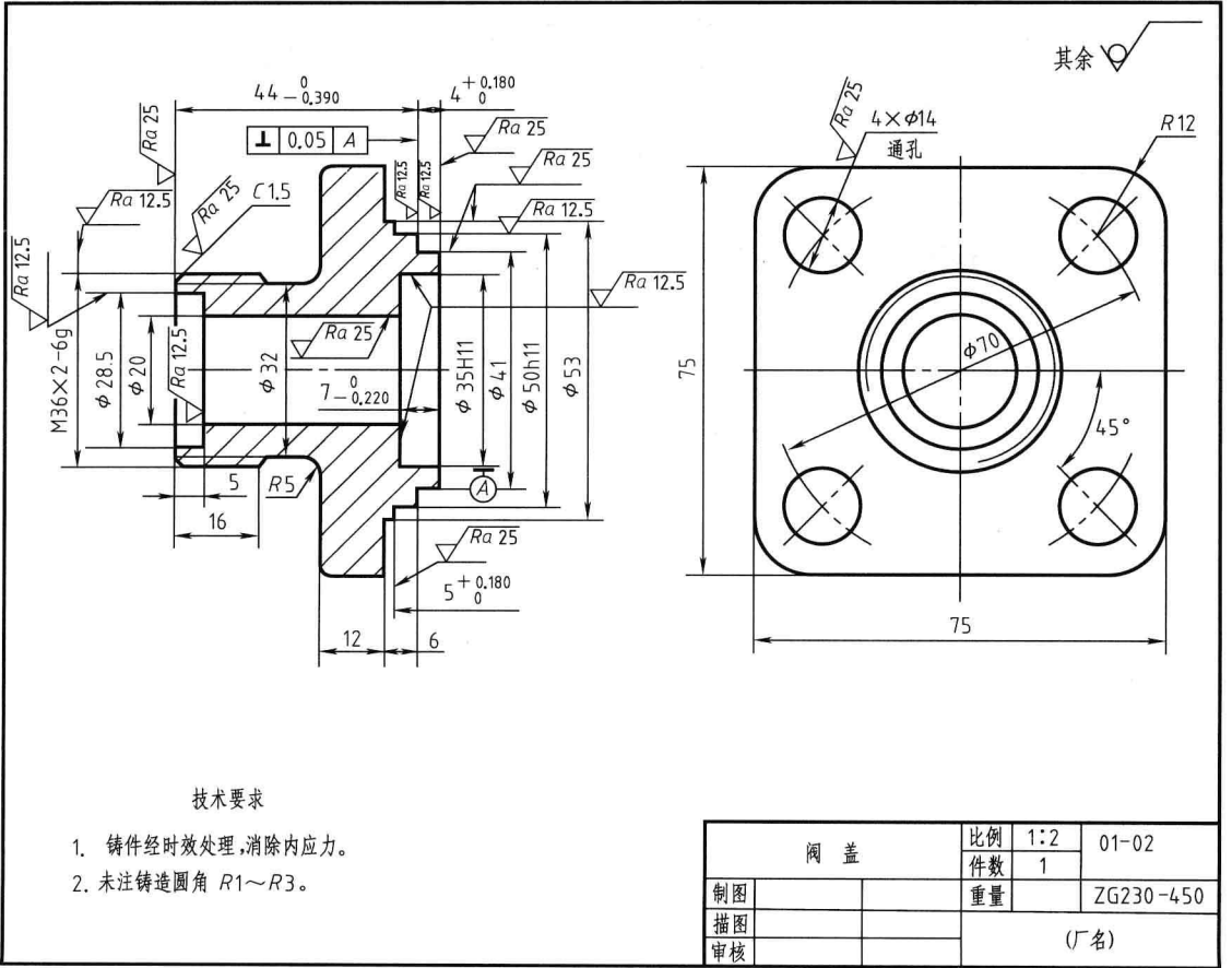
图 1-1 阀盖零件图
