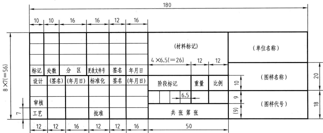
图 1-3 标题栏的格式及尺寸
