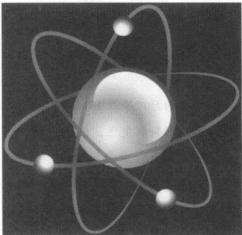
原子模型图
