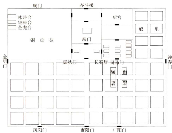
图1-15 曹魏邺城平面布局图
