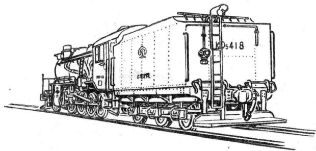
KD 5 型机车 (调度用)
