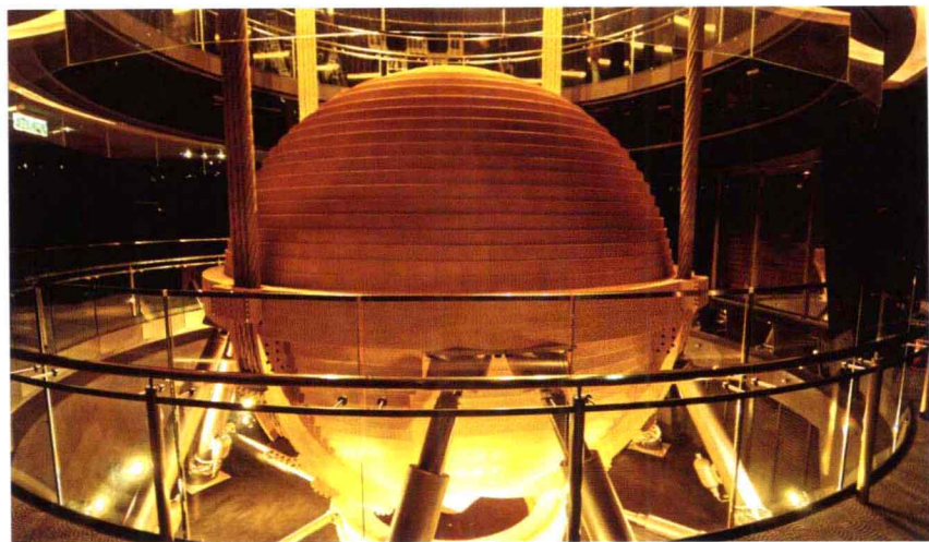
台北101大楼88~92楼层挂置的世界最大的阻尼器。
