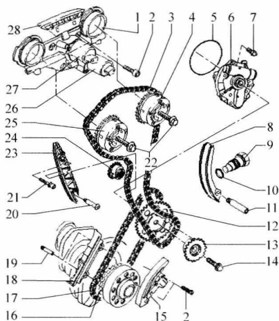
图 1-1 Q7 轿车 3.6L BHK 发动机正时链条部件识别
