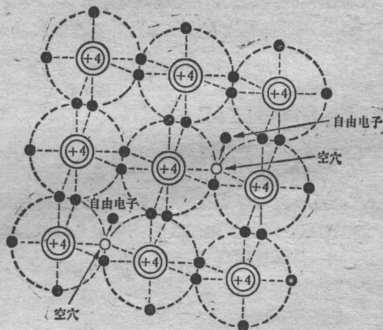
图 1-4 热运动产生的电子-空穴对
