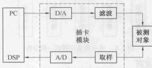
图 1.3 虚拟仪器
