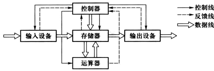
图 1.1 以存储器为中心的计算机结构
