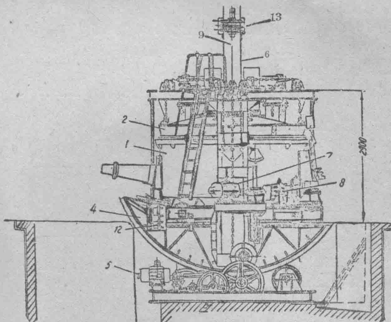
图 2—1 5 吨炉頂装料式电炉
