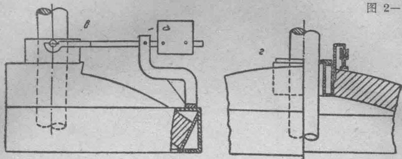
图 2—7 密封圈装置
