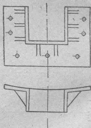
图 2-10 装料門門框
