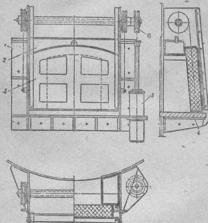
图 2-9 电弧炉的装料門
