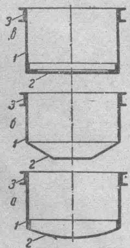
图 2—2 电弧炉的炉壳 1—圆筒形炉身；2—炉壳底；3—加固圈
