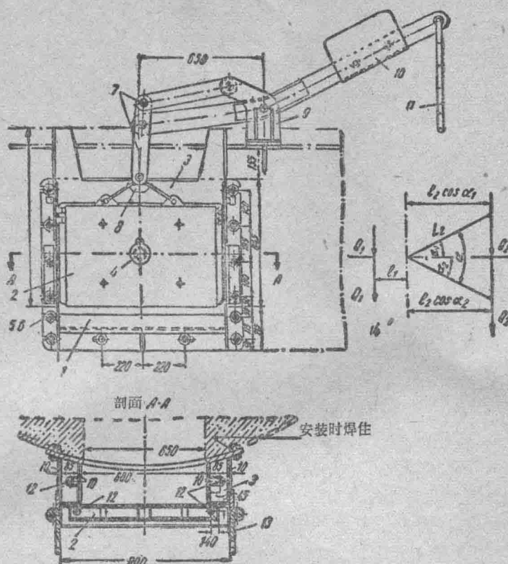
图 2-11 5吨电弧炉装料門的结构
