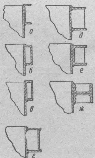
图 2—3 炉壳加固圈
