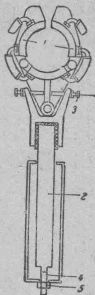
图 2-13 鉗式电极把持器的装置略图
