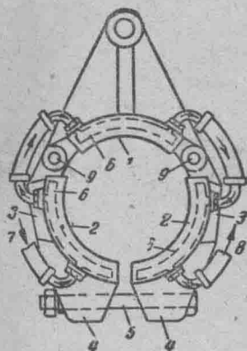
图 2-12 鉗式电极把持器
