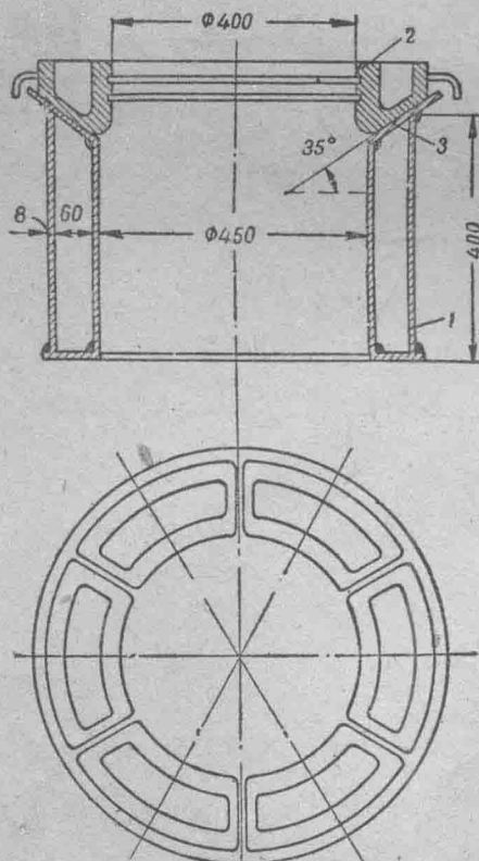
图 2—6 別列耶夫式电极密封圈
