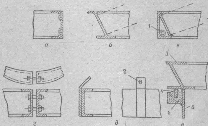
图2—5 炉頂圈的断面形状
