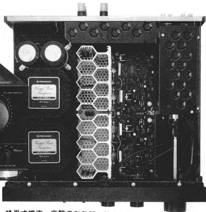
蜂巢式機座、底盤及散熱器、防止共振改善音質
