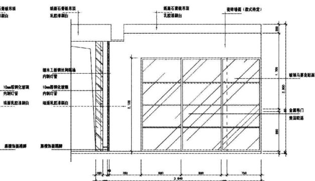
◆ 厨房B 立面图
