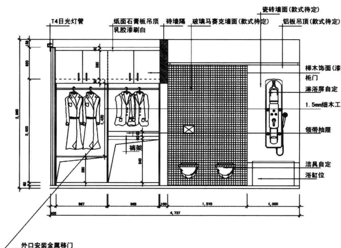
◆ 主卧室卫浴衣帽间B 立面图
