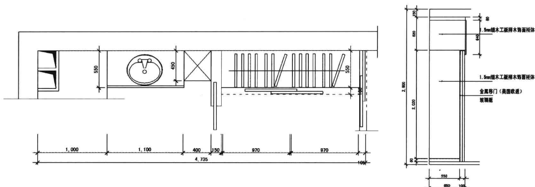
◆ 衣帽间衣柜D 剖面图
