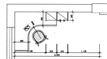
◆ 衣帽间衣柜D 内部结构
