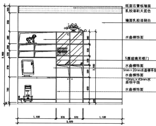
◆ 女孩房B 立面图
