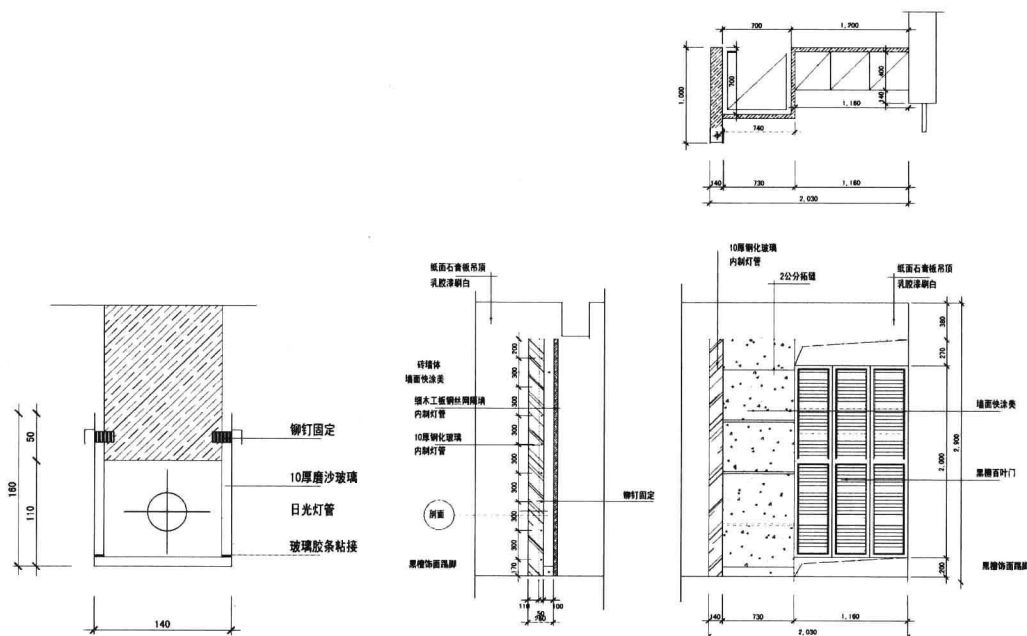
◆ 玄关立面图
