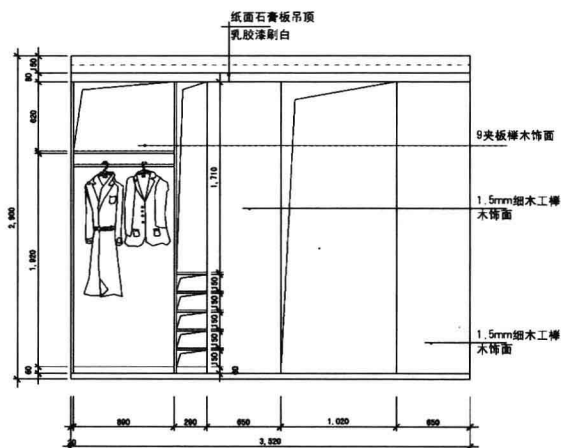
◆ 进门C (衣柜内部) 立面图
