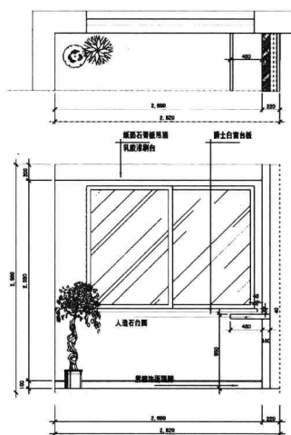
◆ 餐厅C 立面图
