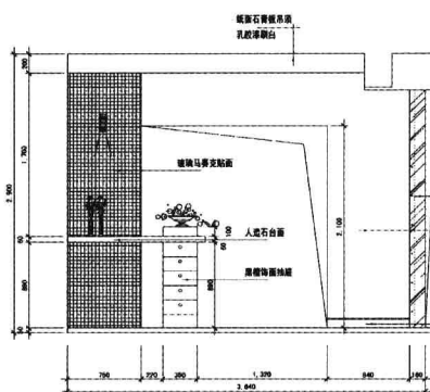
◆ 餐厅D 立面图
