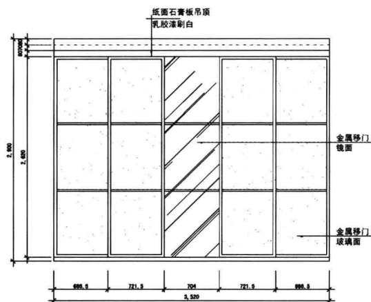
◆ 主卧室C 立面图
