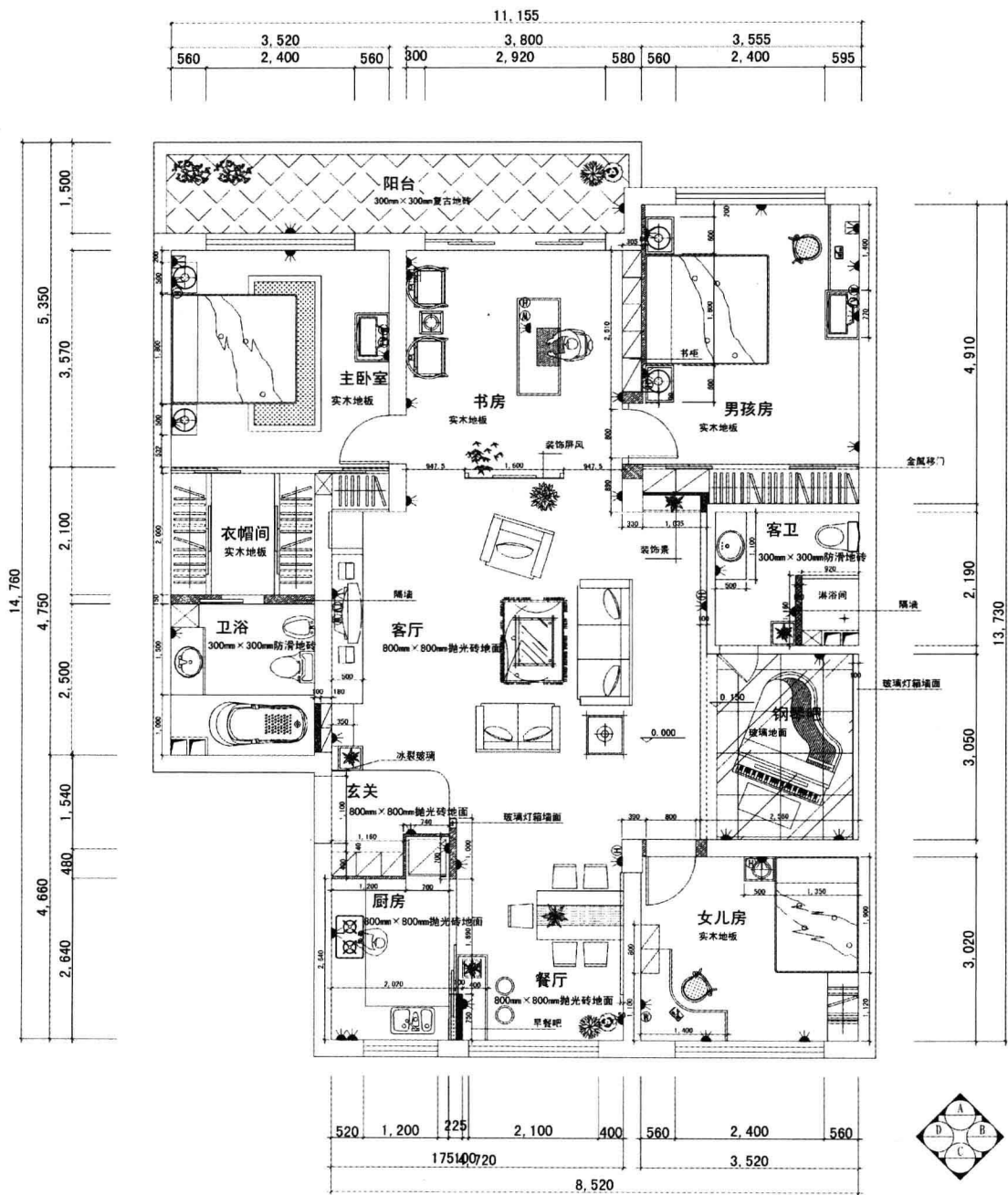
◆ 弱电插座布置图
