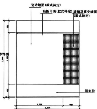
◆ 主卧室卫浴C 立面图
