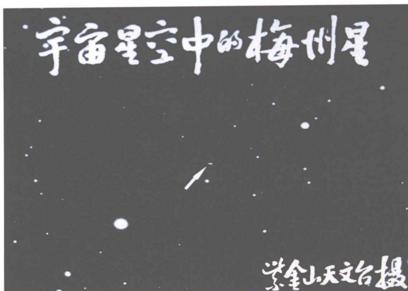
(3239) 梅州星 照片說明 照片中箭頭所指的短條狀星像為在宇宙星空中不斷移動的(3239)梅州星(紫金山天文臺用口徑40厘米的雙筒望遠鏡拍攝,露光60分鐘),周圍點狀星像均為恆星。
