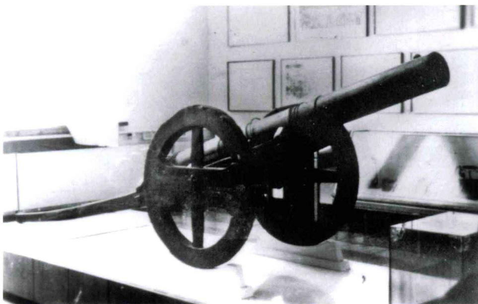
1928年琼崖红军军械厂在乐会县四区制造的荔枝炮。
