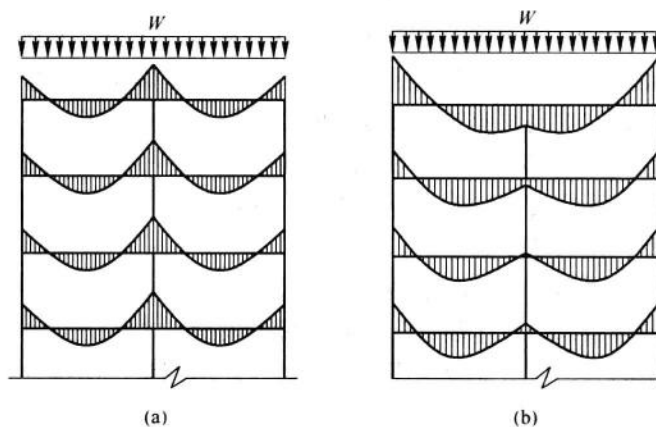
图1-7 柱轴向变形对高层框架梁弯矩分布的影响
