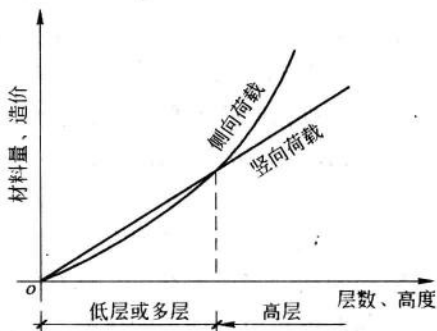
图 1-8 荷载、材料与建筑高度的关系
