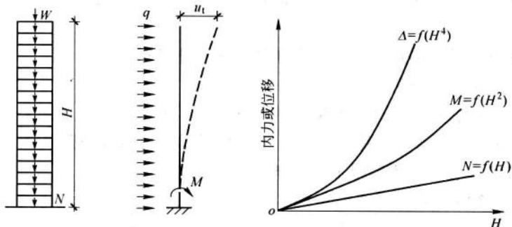
图 1-6 结构内力、位移与高度的关系
