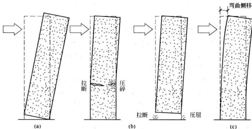
图 1-4 建筑物抗弯曲
