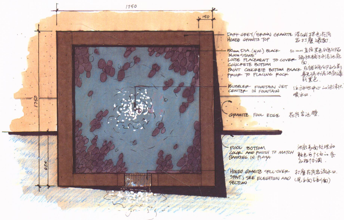
花岗岩喷泉水池平面图
