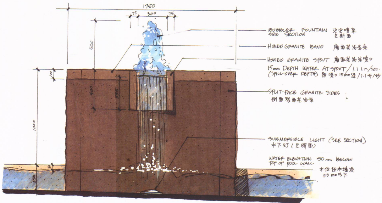
花岗岩喷泉水池立面图
