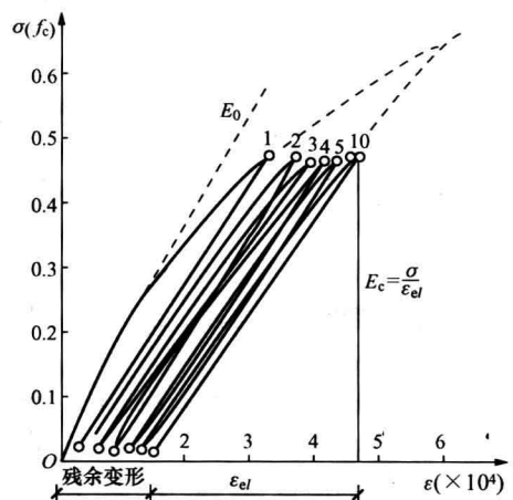
图 1-14 混凝土弹性模量 E_c 的测定方法
