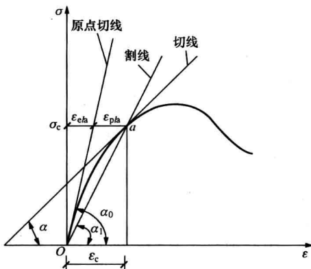
图 1-13 混凝土变形模量的表示方法
