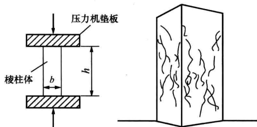
图 1-3 混凝土棱柱体抗压试验
