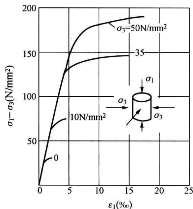
图 1-9 受液压作用的圆柱体试件
