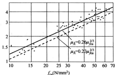
图 1-6 混凝土轴心抗拉强度与立方体抗压强度的关系
