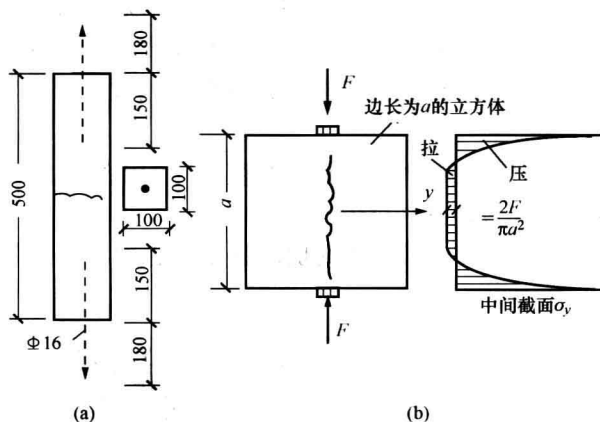
图 1-5 混凝土抗拉强度试验示意图
