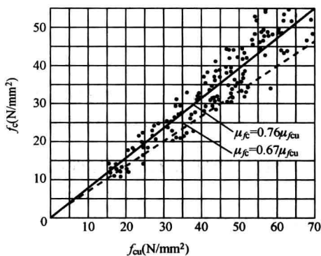
图1-4 轴心抗压强度与立方体抗压强度的关系
