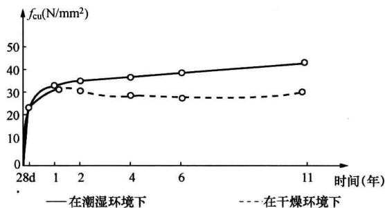
图 1-2 混凝土强度随龄期增长曲线
