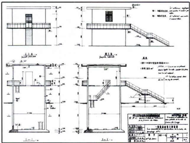
刚果韦索市给水工程——级泵房建筑图
