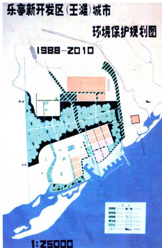
乐亭新开发区(王滩)城市环境保护规划图
