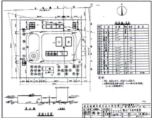
迁安县城给水工程——配水厂平面布置图
