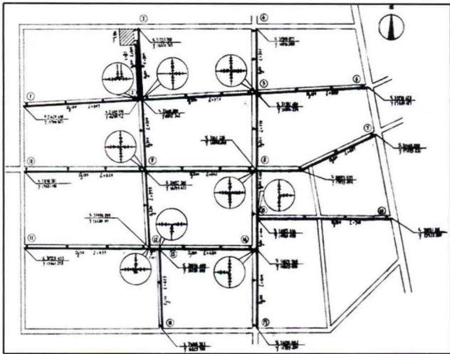
迁安县城给水工程——管网平面布置图 (1982年)
