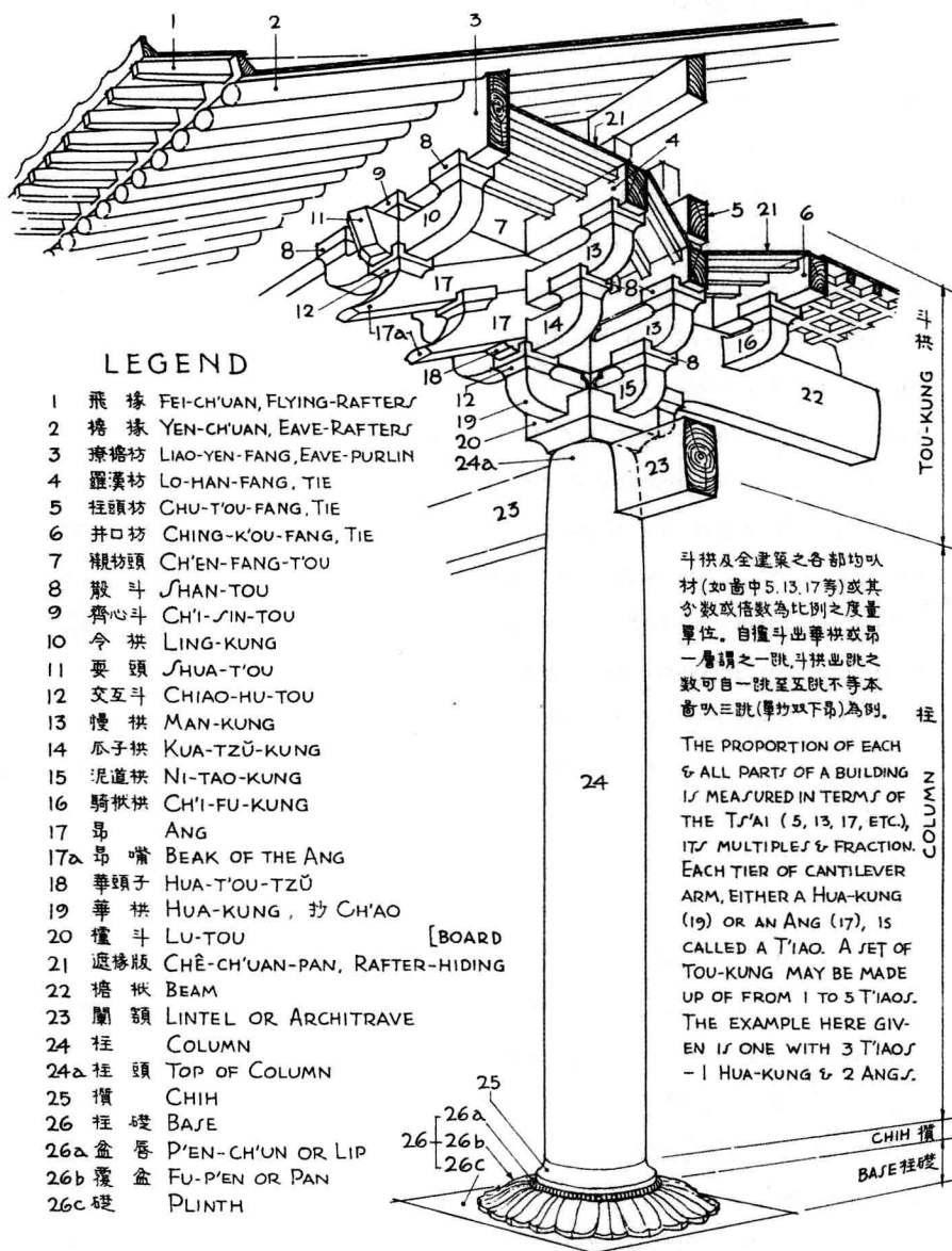
中國建築之“ORDER”·斗拱, 檐枋, 柱礎, 柱礎 THE CHINESE “ORDER”
