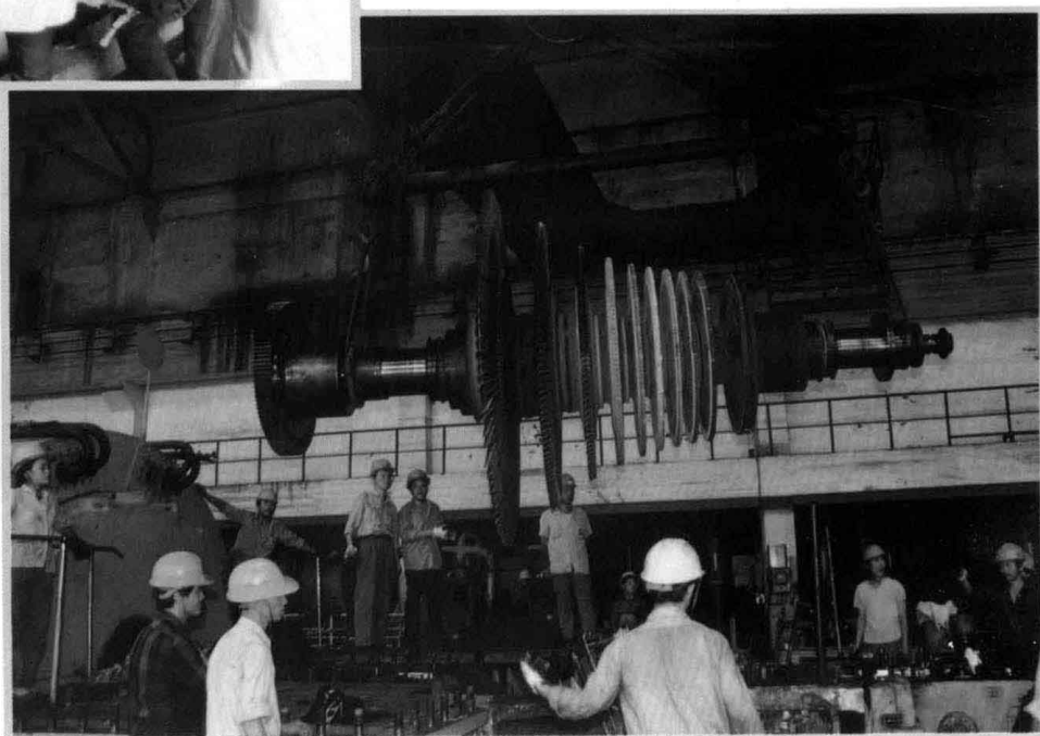
大修中起吊汽轮机转子。
