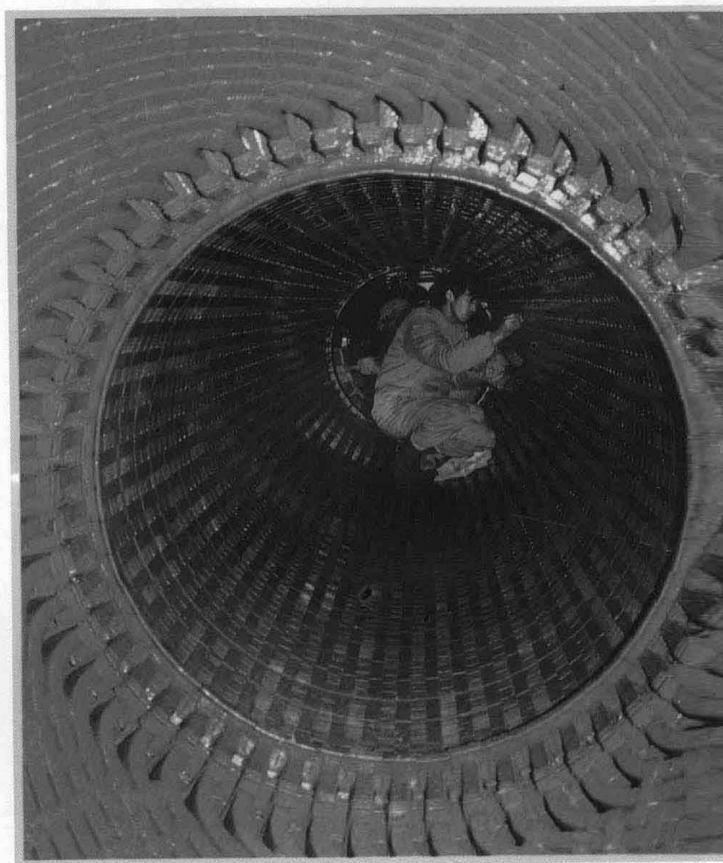
检查20万千瓦发电机静子。 韩虹杰 摄
