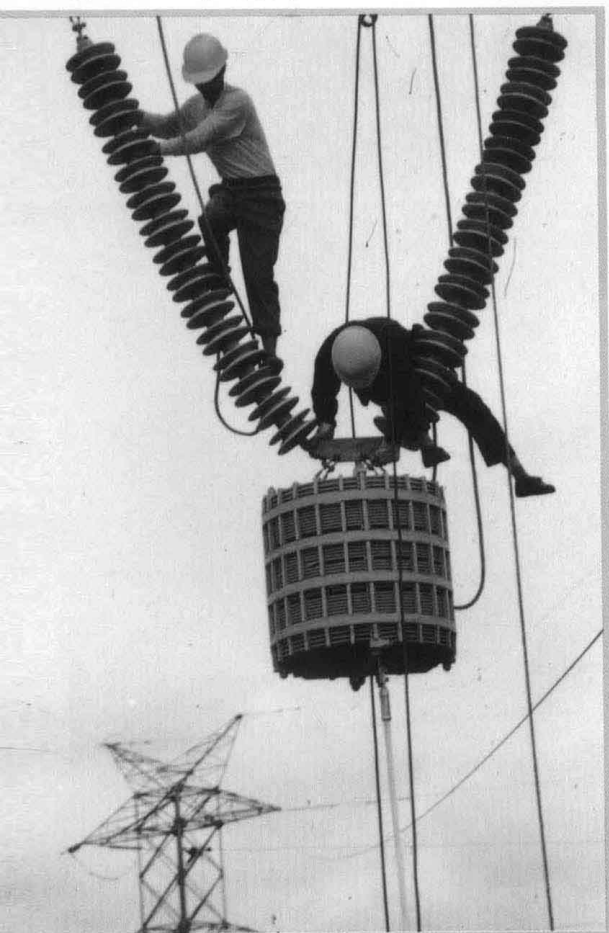
安装220千伏高压输电线路阻波器 (1995年3月)。 韩虹杰 摄
