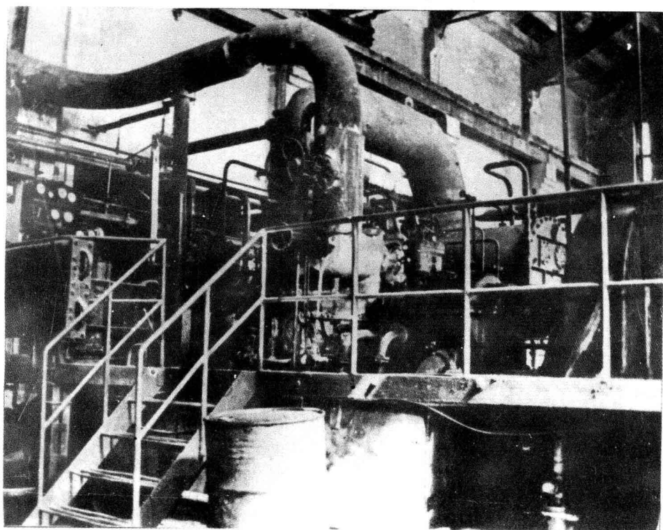
25 周口电厂1500吨发电机组汽轮机部分
