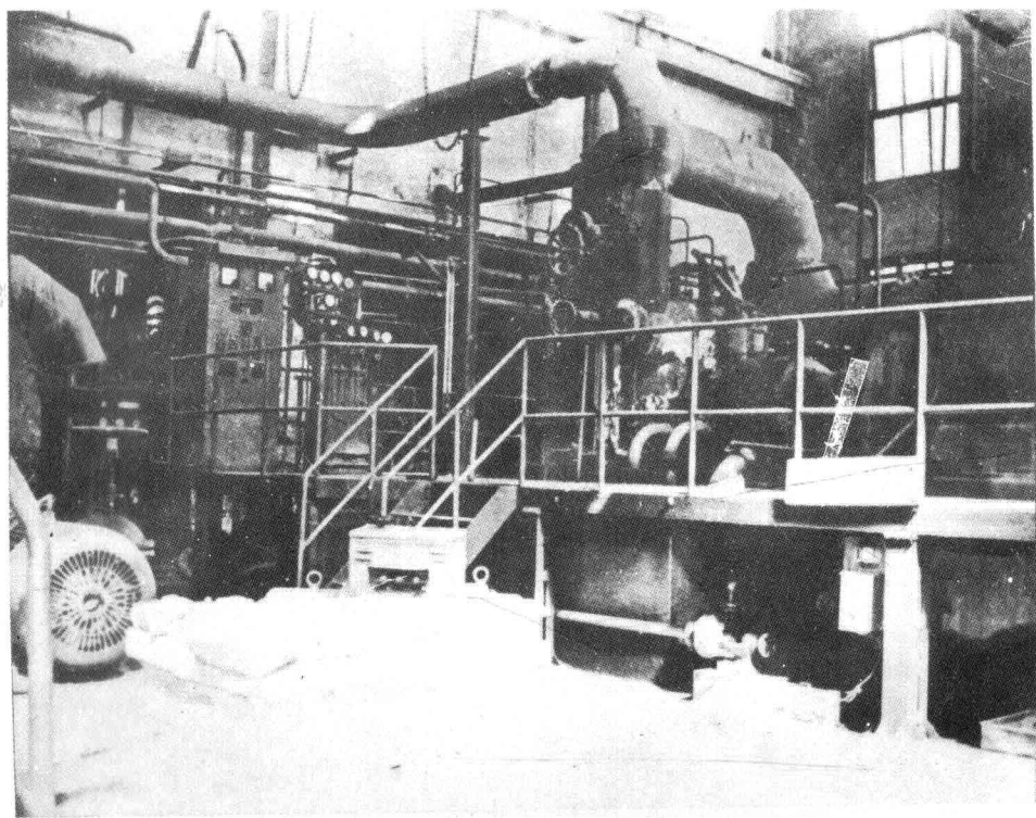
26 周口电厂 2 \times 1500 汽轮发电机组
