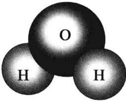
图 2-1 水分子的结构
