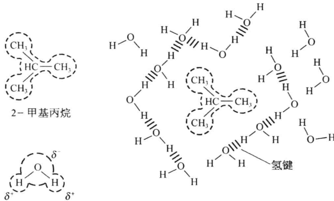
图 2-3 疏水分子在水溶液中的存在形式
