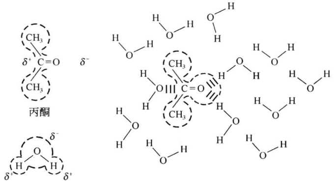
图 2-2 亲水分子在水溶液中的存在形式
